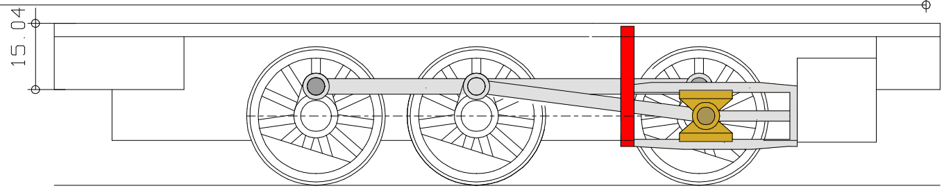
Ansicht Antrieb rechte Lokseite
